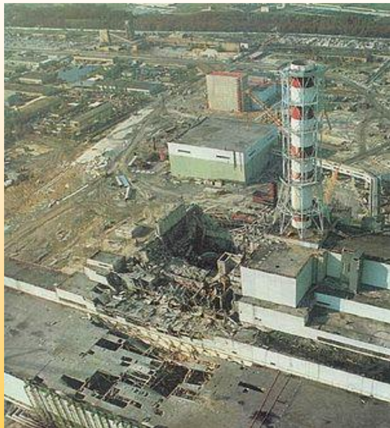
Четвертий енергоблок ЧАЕС після аварії
